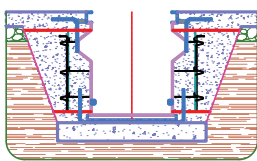
Dobbeltlag - ved ustabile grunnforhold
