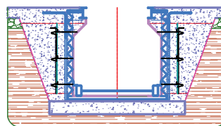
Dobbeltlag - ved ustabile grunnforhold
