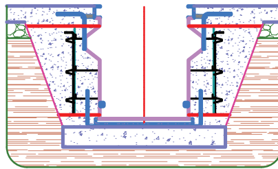
Double peau pour sols de mauvaise qualité
